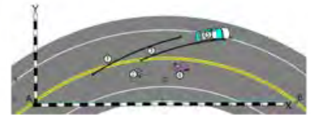
Imagen 97. Ejemplo de fijación de accidente en curva con el método de coordenadas. Fuente: archivo académico software EDGE FX.
