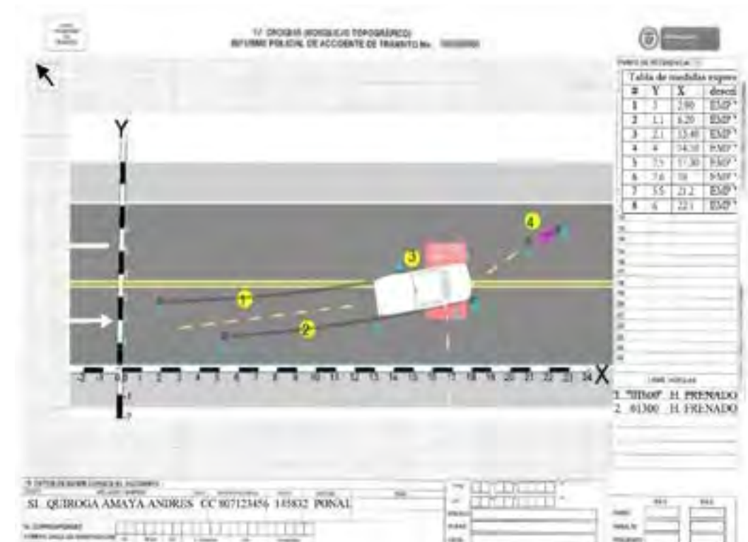
Imagen 91. Ejemplo de la fijación topográfica con el método de coordenadas cartesianas. Fuente: Archivo ESEVI software EDGE FX.
