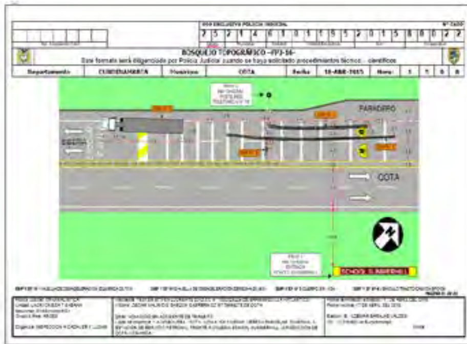
Imagen 93. Ejemplo de un dibujo topográfico fijado y acotado método ortogonal. Fuente: Archivo Subintendente Ildemar Barajas Valdés, LACRI DITRA.
