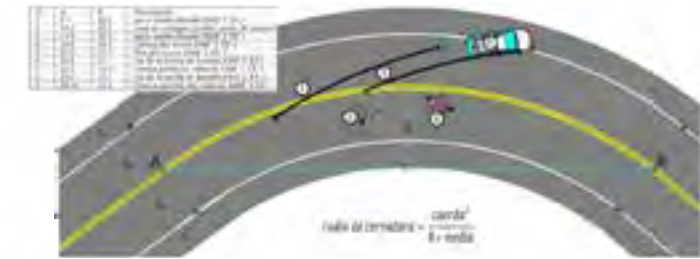
Imagen 96. Ejemplo de fijación de accidente en curva con el método de triangulación. Fuente: archivo académico software EDGE FX.
